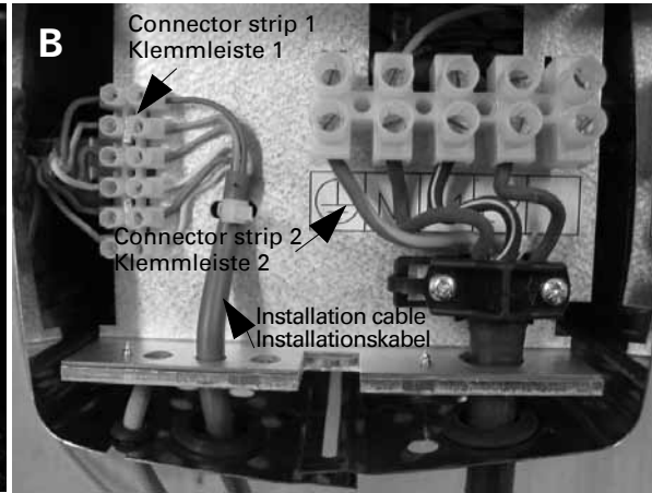
Figure 10 A and B. 2-phase electrical connections of the heater Abbildung 10 A und B. 2-Phasen-Elektrische Anschlüsse des Saunaofens
