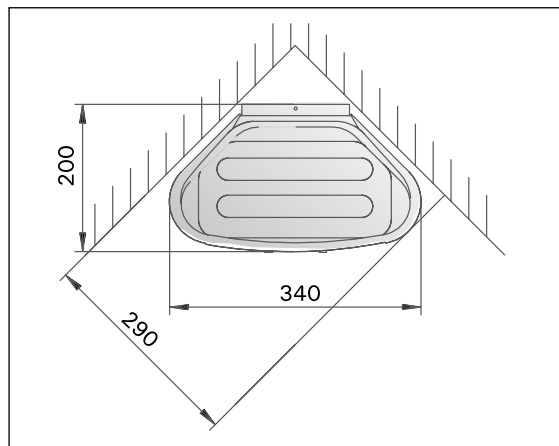
Figure 4. Dimensions of heater Abbildung 4. Maße des Ofens
