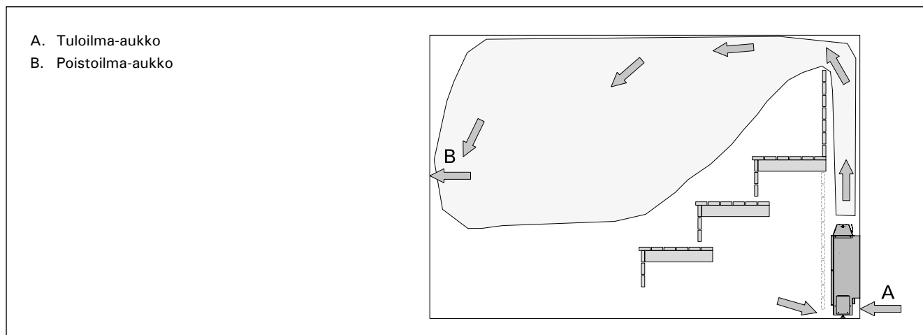
Figure 3. Saunahuoneen ilmanvaihto
